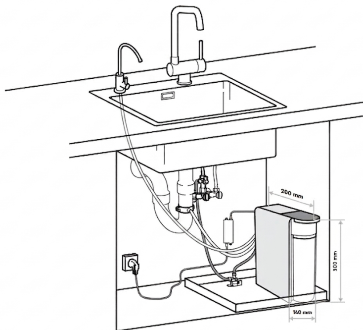
Anschlussübersicht unter der Spüle
